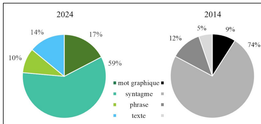
Figure 48 : Complexité morphosyntaxique
